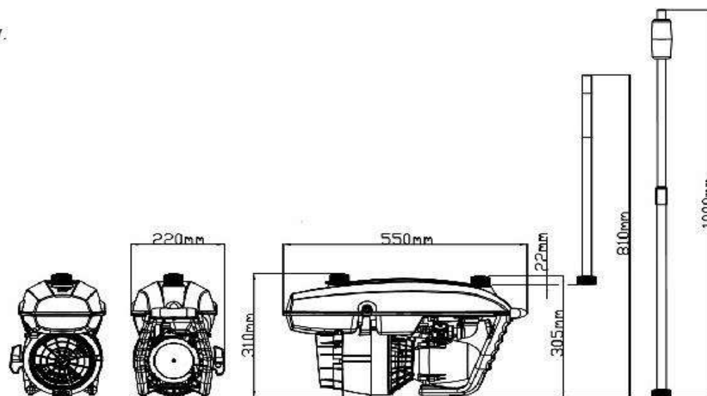
DIMENSIONI DI INGOMBRO - OVERALL SIZES
